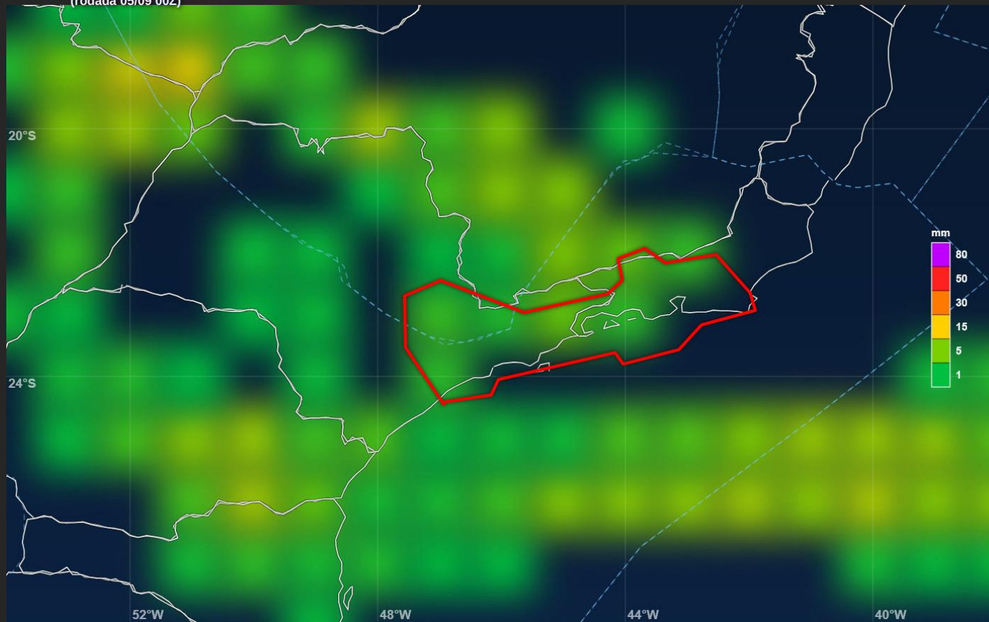
Modelagem ECMWF — precipitação prevista (pico) · 2000 UTC 05/09 (rodada 05/09 00Z)
